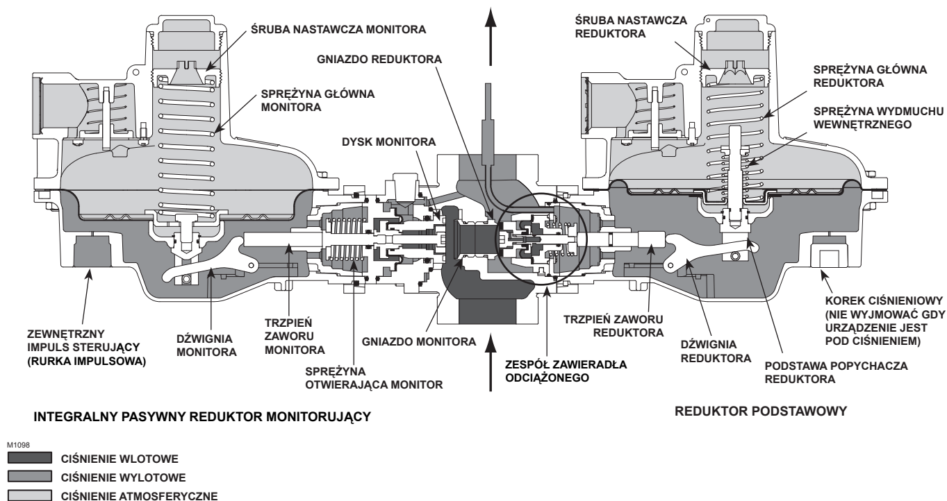
Rysunek 5. Typ CSB403IT reduktor podstawowy z impulsem wewnętrznym oraz z monitorem integralnym z impulsem zewnętrznym - schemat działania
