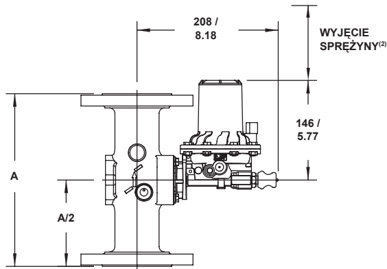
MODUŁ ZAWORU SZYBKO ZAMYKAJĄCEGO
