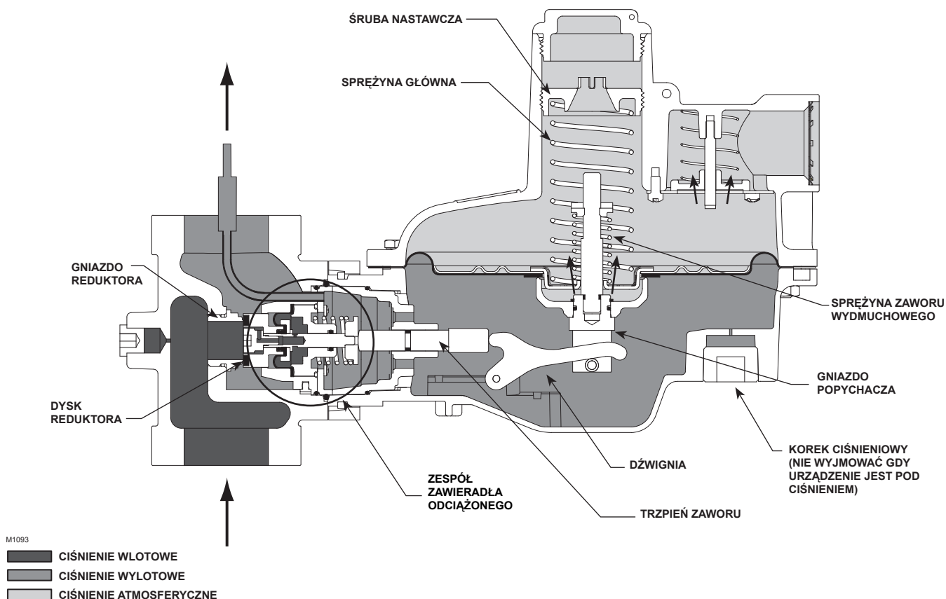
Rysunek 4. Seria CSB400 z wewnętrznym impulsem i zaworem wydechowym - schemat działania
