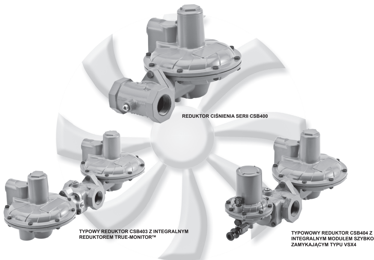
Rysunek 1. Typowe reduktory ciśnienia Serii CSB400
