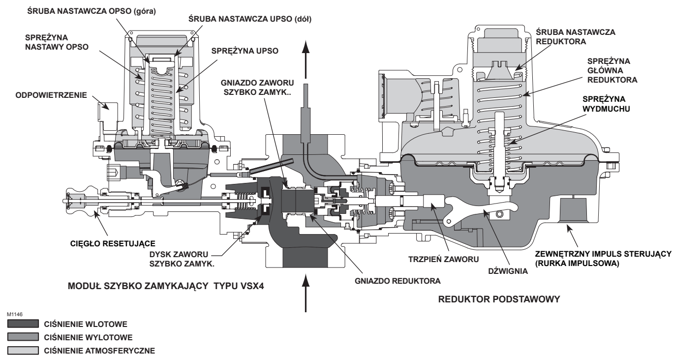
Rysunek 6. Typ CSB404ET reduktor oraz zawór szybko zamykający z impulsem zewnętrznym - schemat działania
