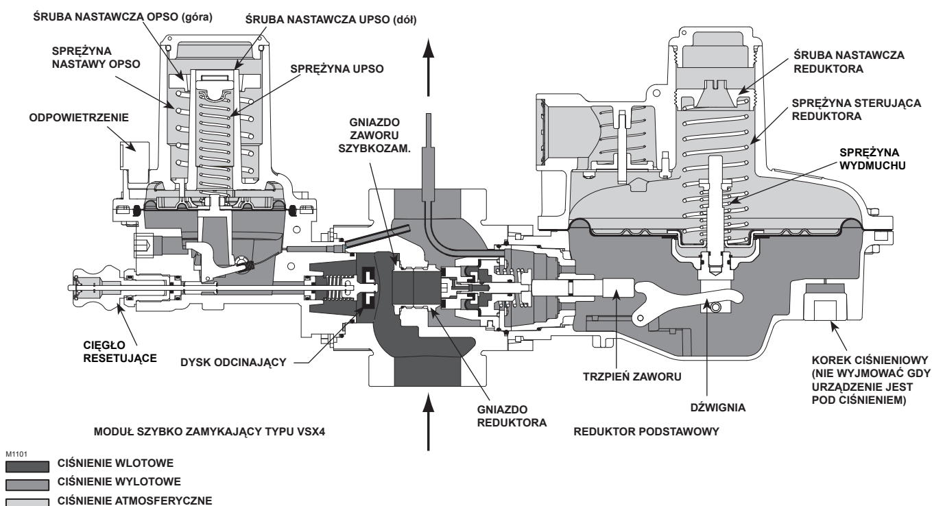
Rysunek 7. Typ CSB404IT reduktor z impulsem wewnętrznym oraz zawór szybko zamykający z impulsem zewnętrznym - schemat działania
