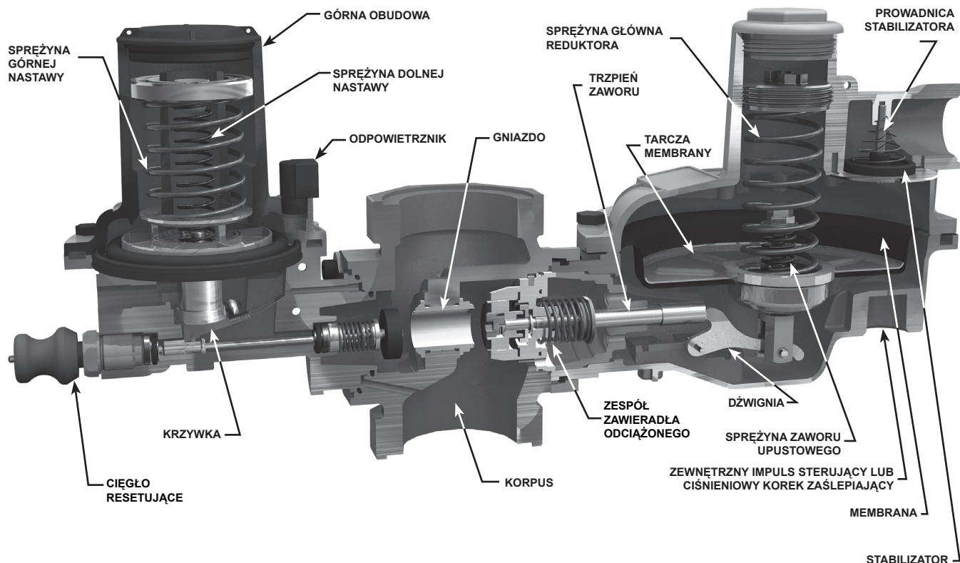
Rysunek 2. Przekrój reduktora Typu CSB404 z zaworem szybko zamykającym Typu VSX4
