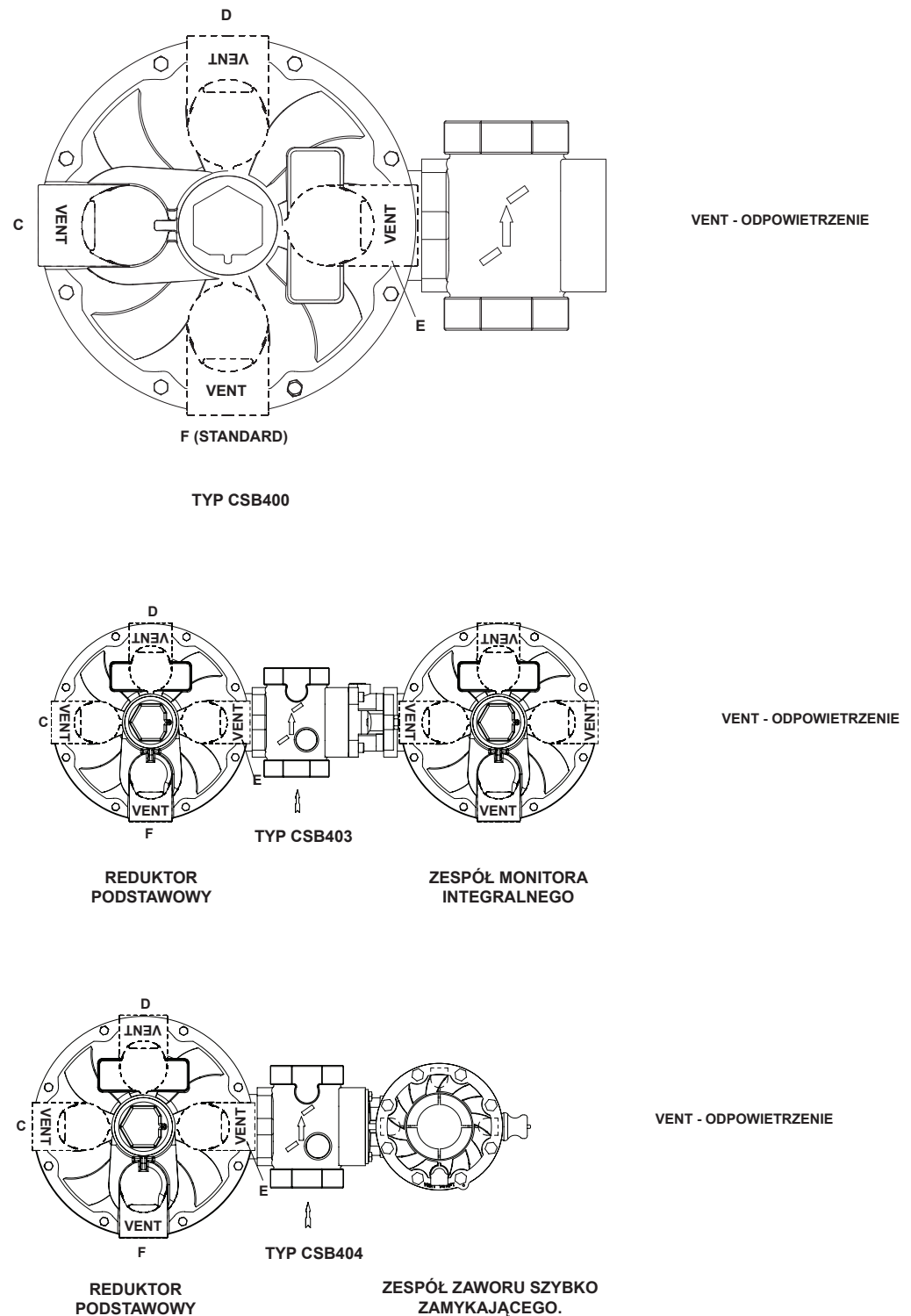
Rysunek 8. Typy CSB400, CSB403 i CSB404 odpowietrzenie obudowy sprężyny i orientacja korpusu
