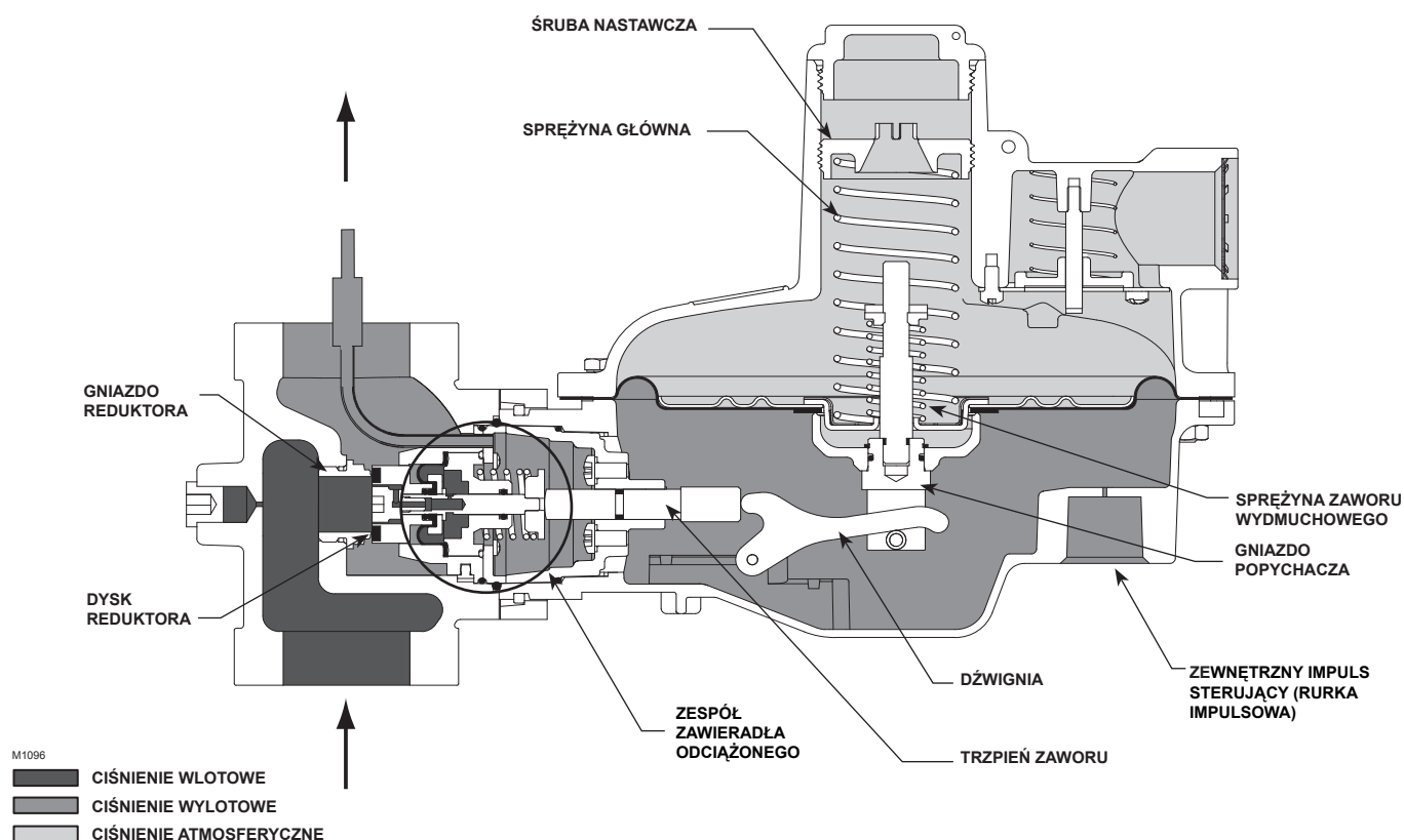
Rysunek 3. Seria CSB400 z zewnętrznym impulsem i zaworem wydechowym - schemat działania
