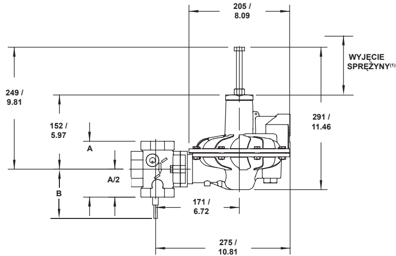
REDUKTOR PODSTAWOWY
