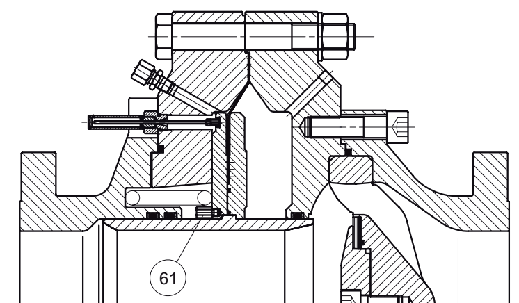
DETAL FL/150 ANSI 300-600
