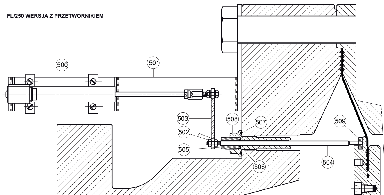
FL/250 WERSJA Z MIKROWYŁĄCZNIKIEM
