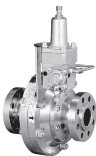
FL - REDUKTOR
