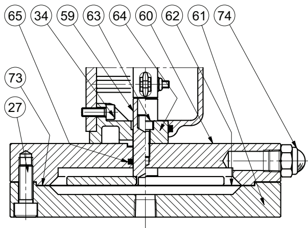
TYP OS/80X-BPA-D
