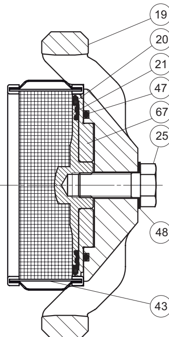
UCHWYT USZCZELKI DN 80, 100, 150
