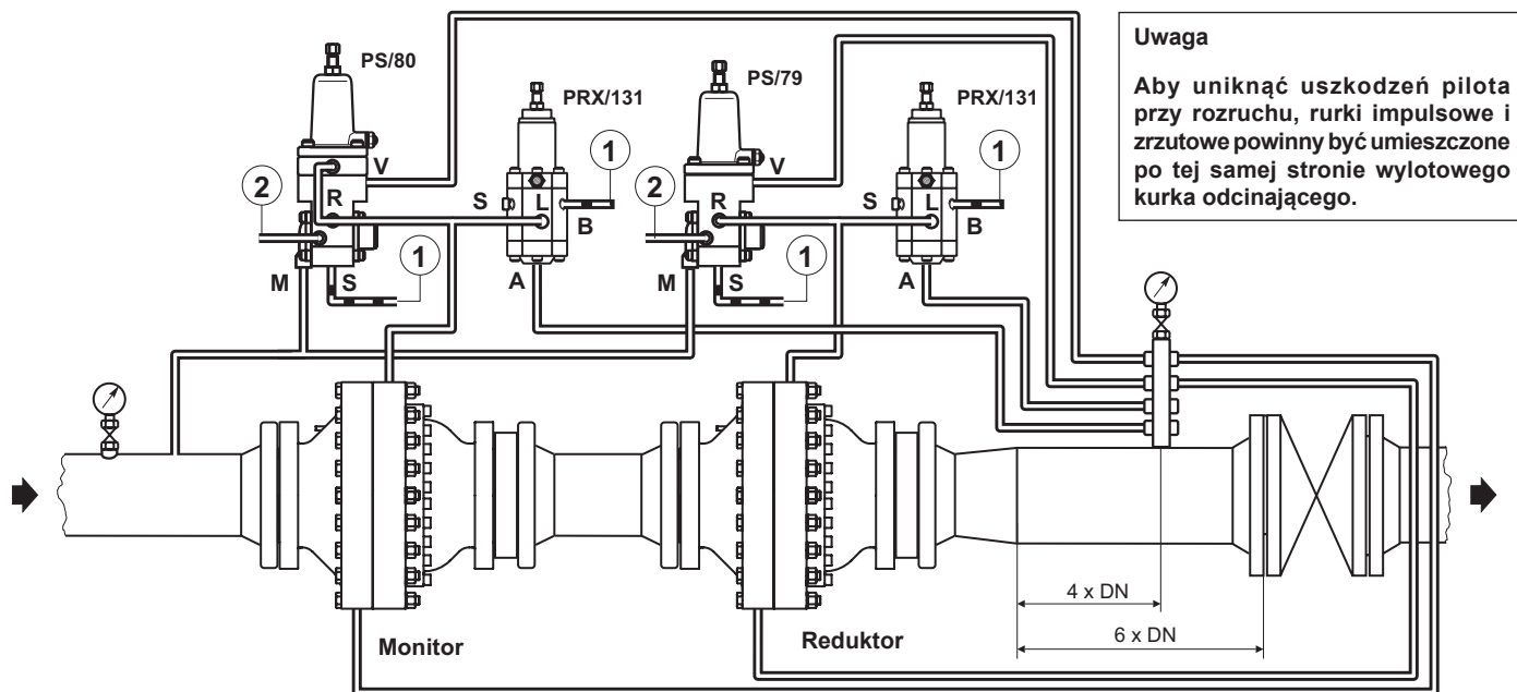
REDUKTOR TYPU FL DN 250 Z PILOTEM PS/79 I PRZYSPIESZACZEM PRX/131, MONITOR Z PILOTEM PS/80 I PRZYSPIESZACZEM PRX/131
