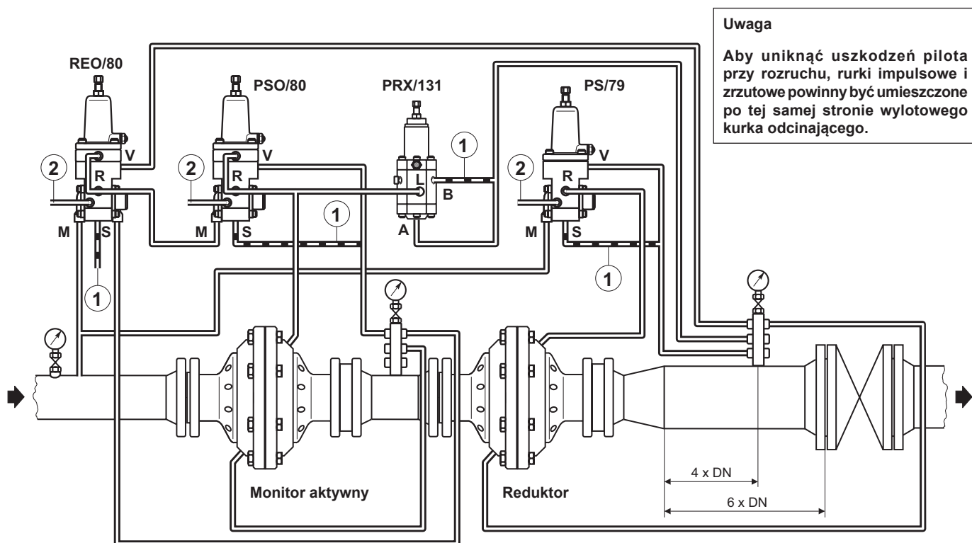
REDUKTOR I MONITOR AKTYWNY TYPU FL Z PILOTEM PS/79, PSO/80, REO/80 I PRZYSPIESZACZEM PRX/131
