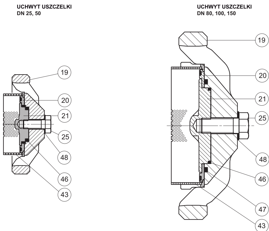
Rysunek 10. Uchwyt uszczelnienia w reduktorze FL DN 25 do DN 150 i reduktorze BFL / MFL DN 25 do DN 100
