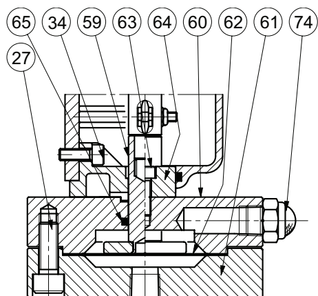
TYP OS/80X-APA-D
