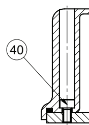
PRZEKRÓJ D-D
