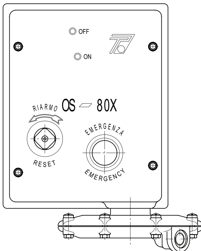
Rysunek 22. Siłownik szybko zamykający serii OS/80X (wersja standardowa)
