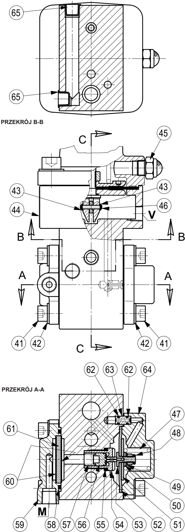
Rysunek 26. Piloty typu PS/79, PS/80, RE/79 i RE/80
