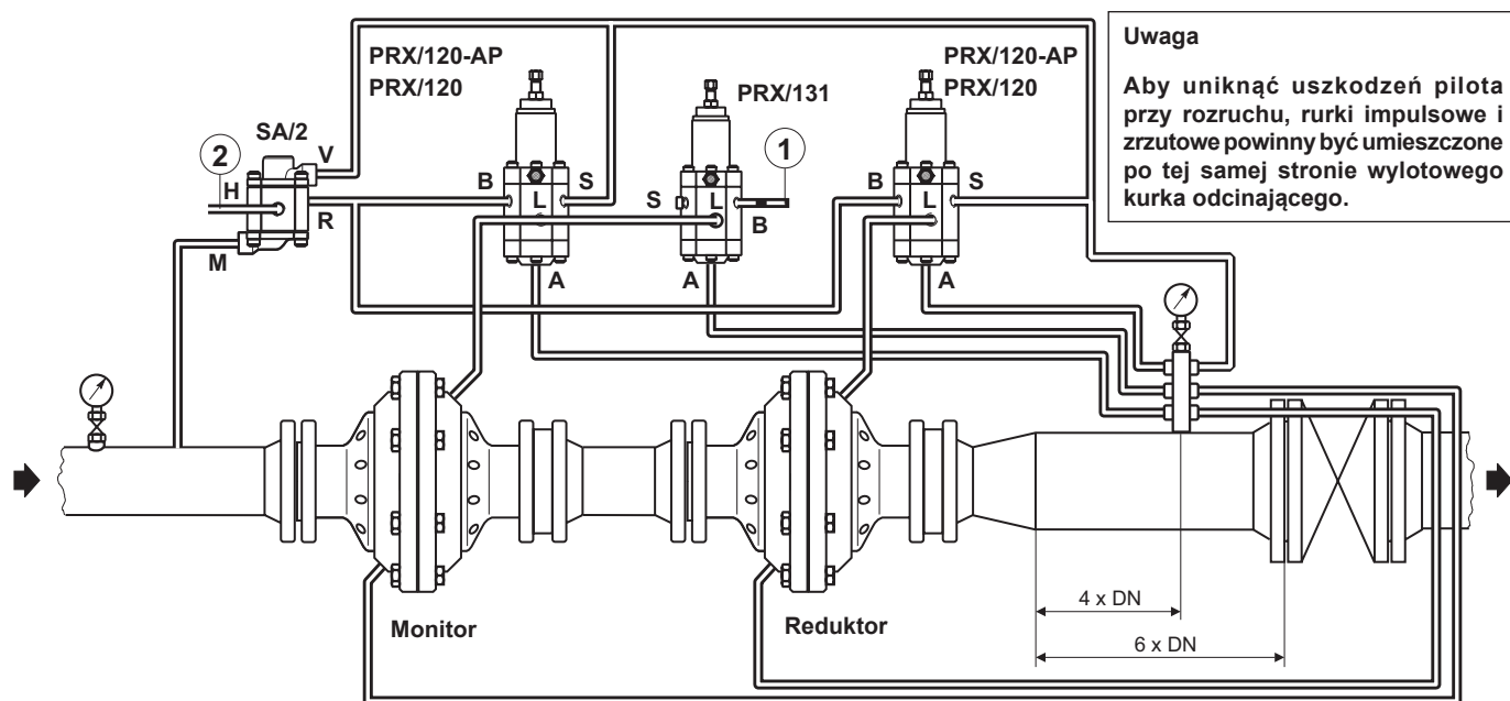
REDUKTOR I MONITOR TYPU FL Z PILOTEM PRX/120 I PRZYSPIESZACZEM PRX/131
