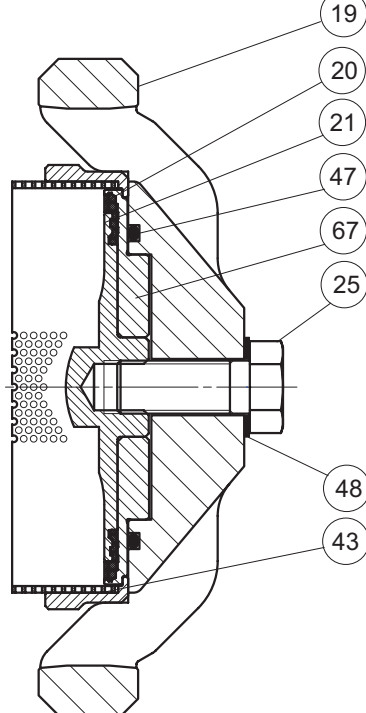
UCHWYT USZCZELKI DN 80, 100, 150
