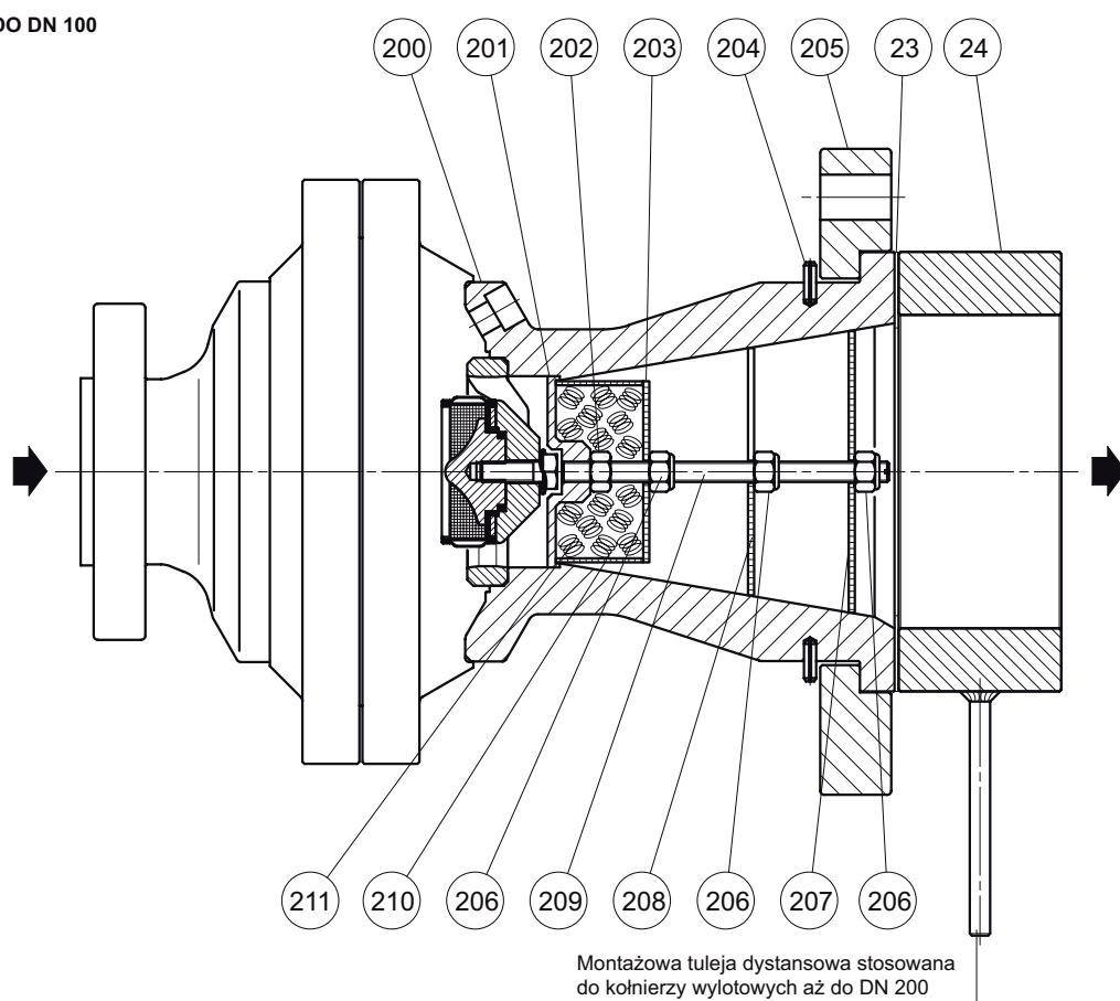
Rysunek 14. Reduktor FL w wersjach: z poszerzonym kołnierzem wylotowym, z tłumikiem SRS i z tłumikiem SRS-R
