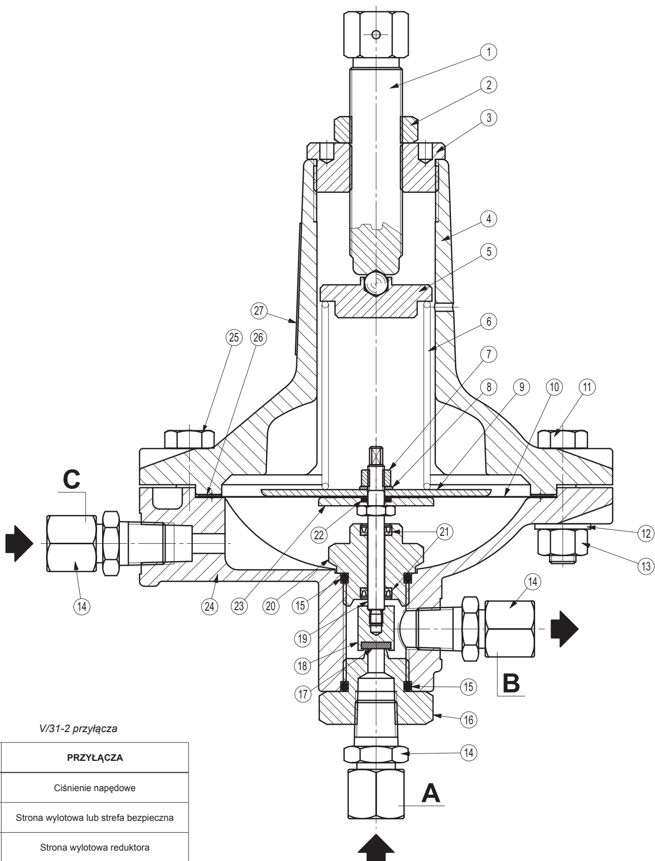
Rysunek 28. Przyspieszacz typu V/31-2
