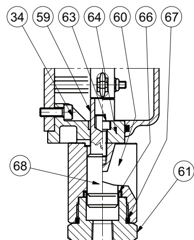
TYP OS/84X
