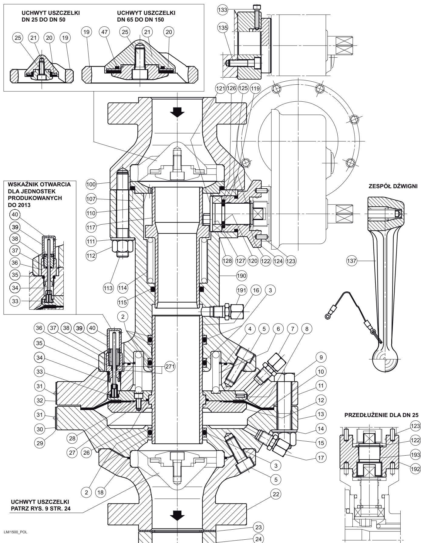
Rysunek 21. BFL - reduktor z zaworem szybko zamykającym
