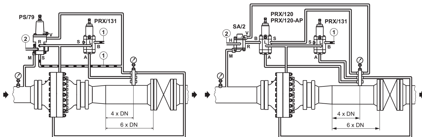
REDUKTOR TYPU FL DN 250 Z PILOTEM PS/79 I PRZYSPIESZACZEM PRX/131
