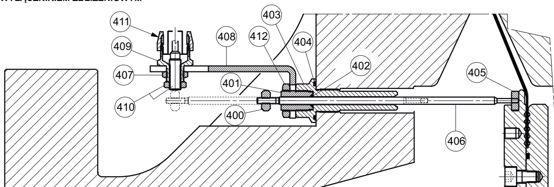
FL/250 WERSJA Z WYŁĄCZNIKIEM ZBLIŻENIOWYM
