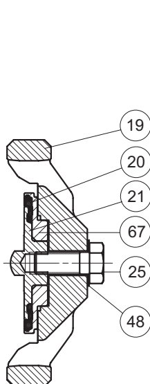
UCHWYT USZCZELKI DN 25, 50
