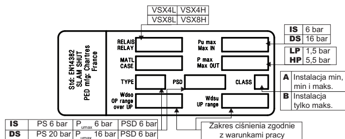
Rysunek 2. Tabliczka znamionowa serii VSX4/VSX8 wg EN 14382
