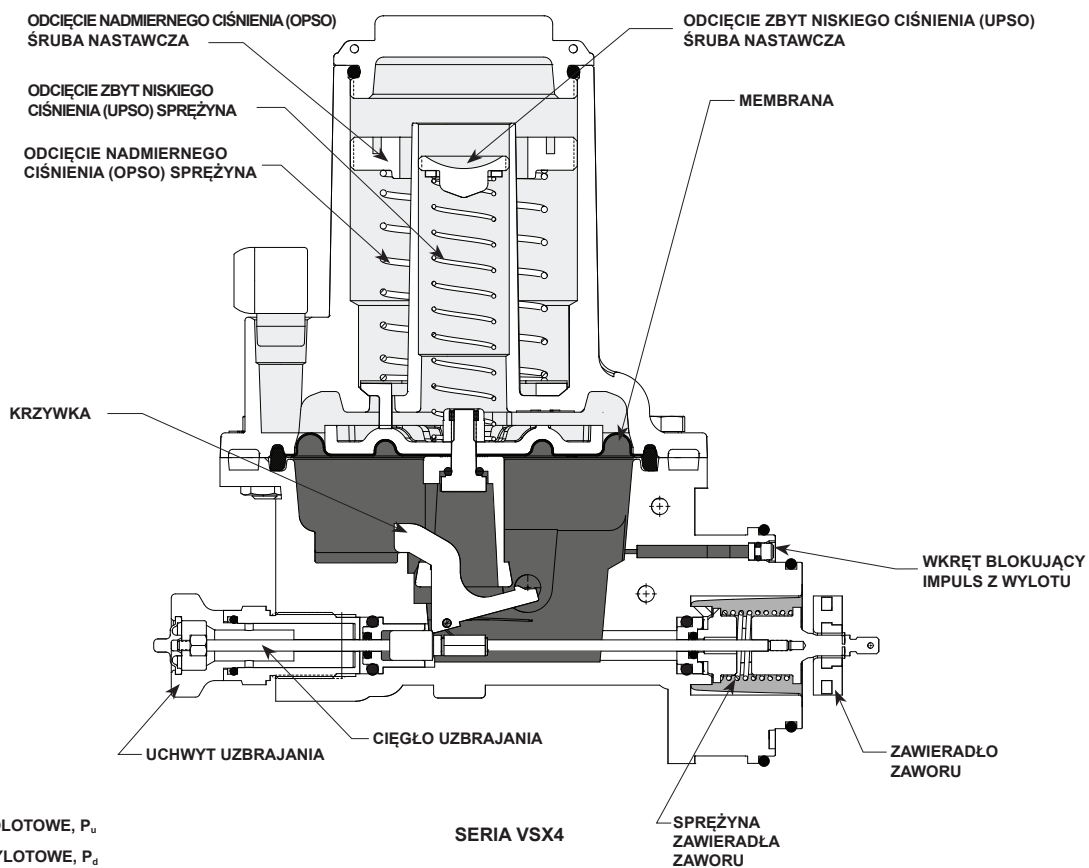
Rysunek 4. Seria VSX4/VSX8 - schemat działania
