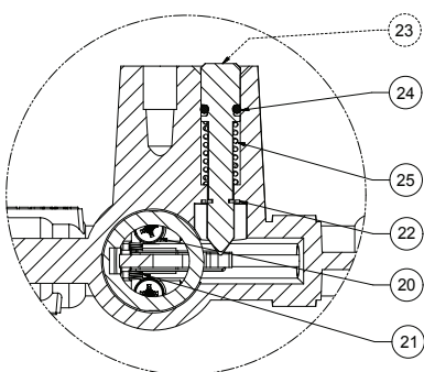
PRZYCIŚK RĘCZNY
