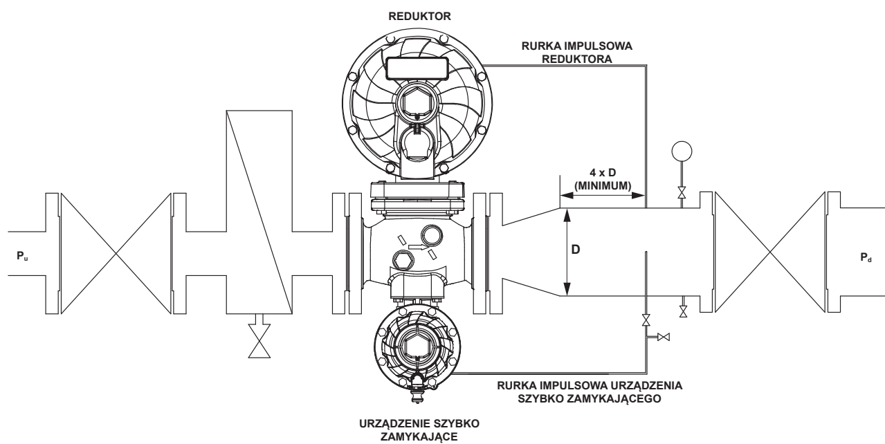
Rysunek 6. Montaż typowego sterownika
