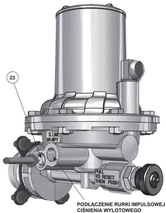
Rysunek 9. Przycisk odcięcia ręcznego (pozycja 23)
